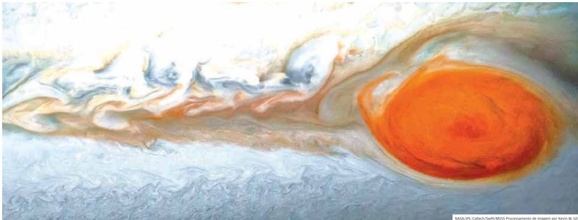
NASA/JPL-Caltech/SwRI/MSSS Processamento de imagem por Kevin M. Gill
